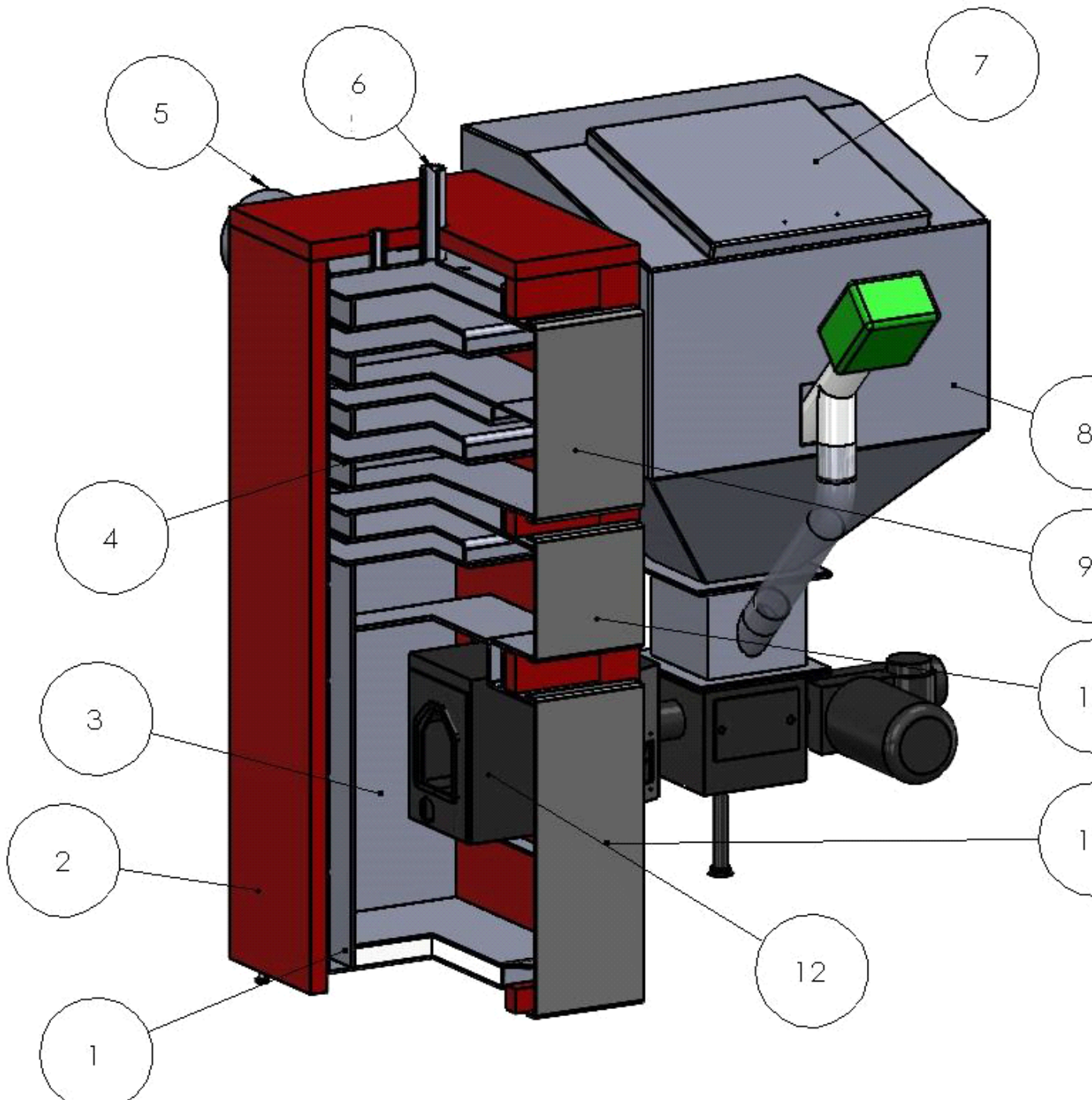
Rys.1. Kocioł "Technix-Pel"
